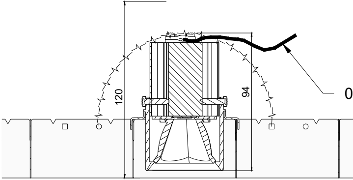
Schnittansicht PUNTEO-J060 - S10 | LVK | Index "a" - 2 x 35°
