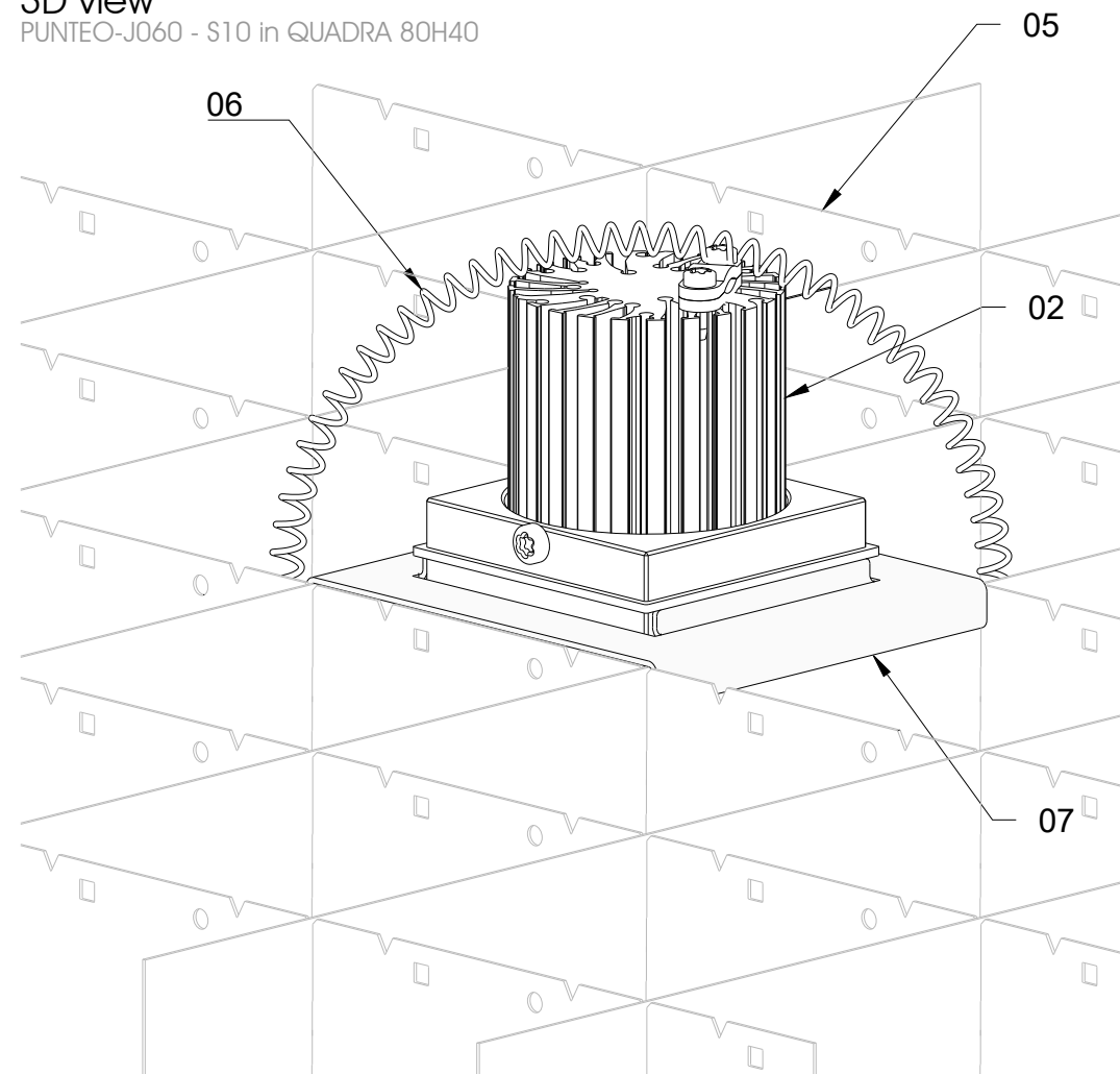
3D view PUNTEO-J060 - S10 in QUADRA 80H40
