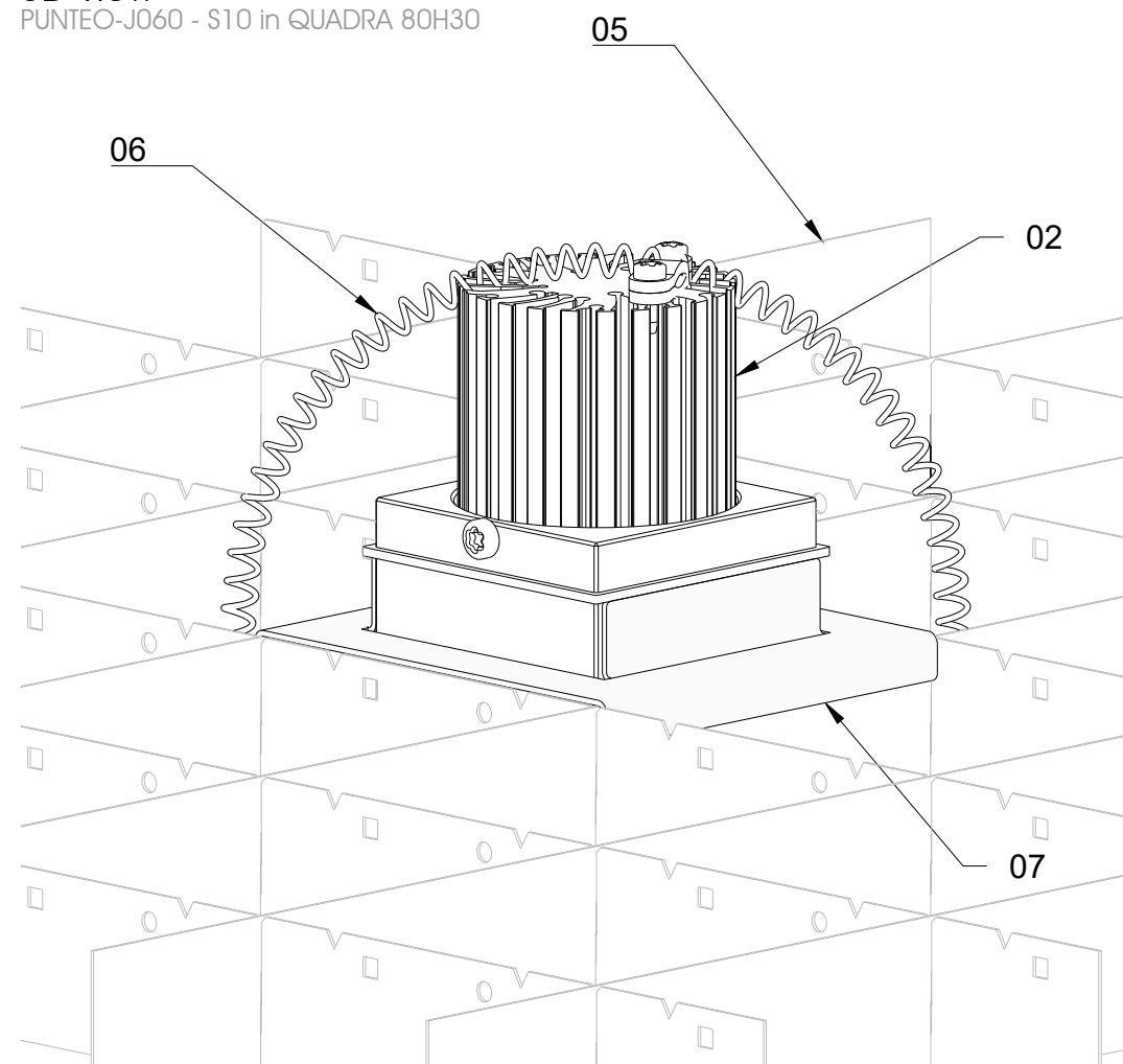
3D view PUNTEO-J060 - S10 in QUADRA 80H30
