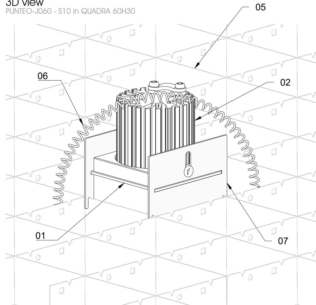
3D view PUNTEO-J060 - S10 in QUADRA 60H30
