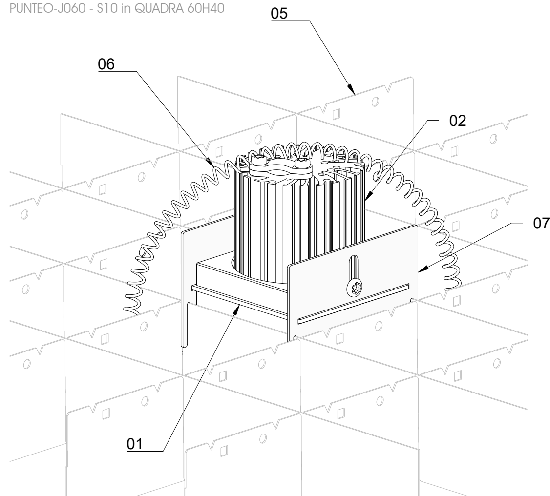
3D view PUNTEO-J060 - S10 in QUADRA 60H40
