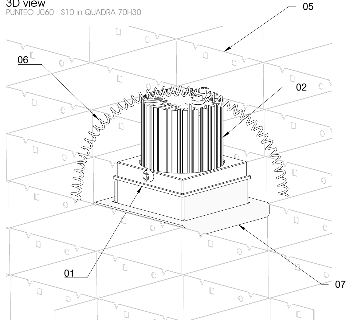
3D view PUNTEO-J060 - S10 in QUADRA 70H30
