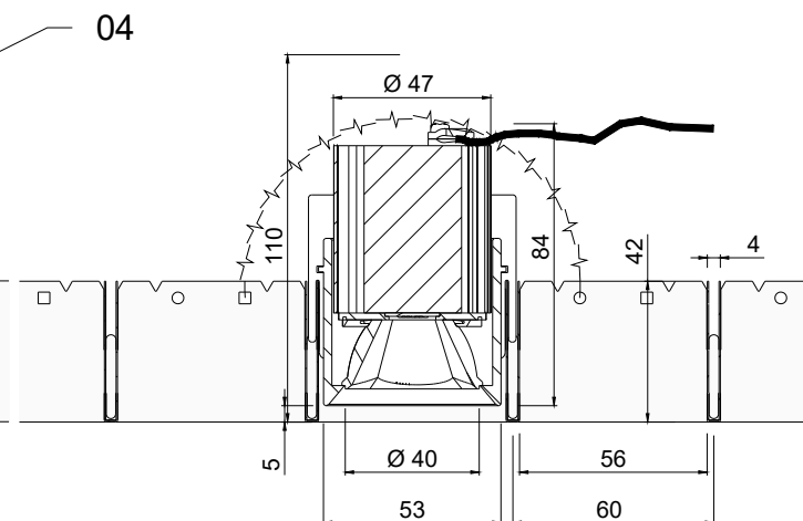
Schnittansicht PUNTEO-J060 - S10 | LVK | Index "b" - 2 x 45°
