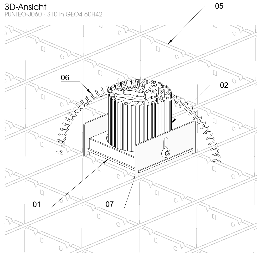
3D-Ansicht PUNTEO-J060 - S10 in GEO4 60H42
