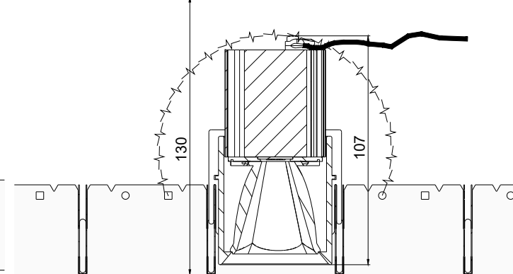
Schnittansicht PUNTEO-J060 - S10 | LVK | Index "c" - 2 x 25°
