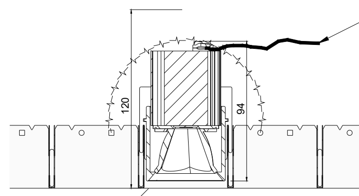
Schnittansicht PUNTEO-J060 - S10 | LVK | Index "a" - 2 x 35°
