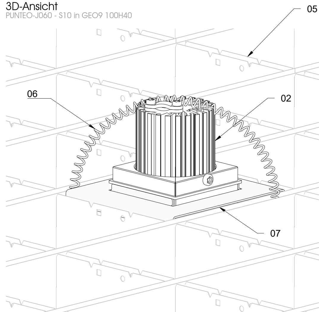
3D-Ansicht PUNTEO-J060 - S10 in GEO9 100H40
