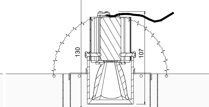
Schnittansicht PUNTEO-J060 - S10 | LVK | Index "c" - 2 x 25°
