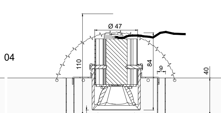
Schnittansicht PUNTEO-J060 - S10 | LVK | Index "b" - 2 x 45°
