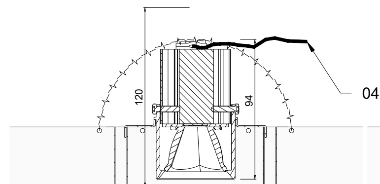
Schnittansicht PUNTEO-J060 - S10 | LVK | Index "a" - 2 x 35°
