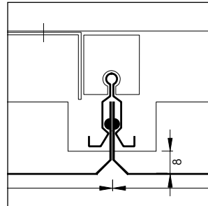
Alternativ mit geringer Abhängenhöhe Alternatively with low suspension height Alternative pour une hauteur de plénum réduite
