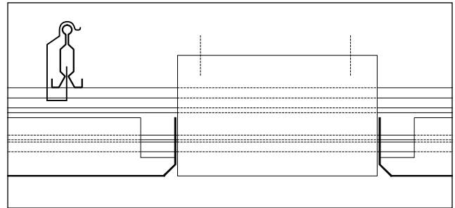
Alternative: Leuchtenabhängung durch Auflegen auf der Decken-UK, Längsseite Alternative: The luminaire is placed on the ceiling suspension, long side Variante: luminaire suspendu sur proteur primaire, côté longueur
