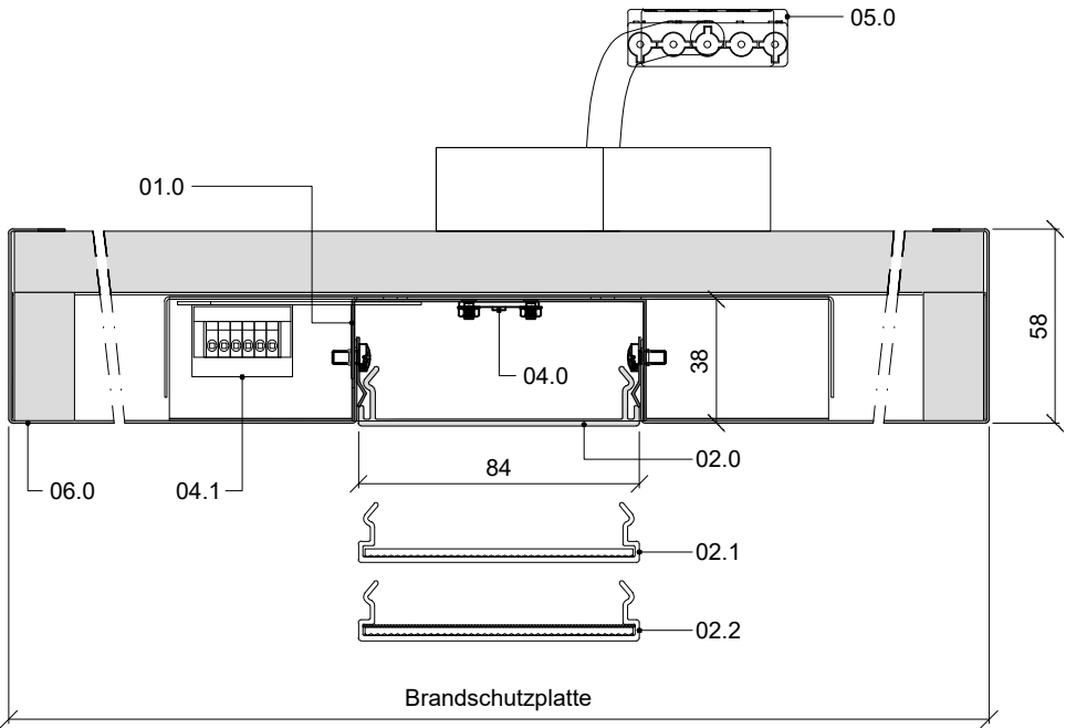
Integration in durlum dur-F30 Brandschutzplatte
