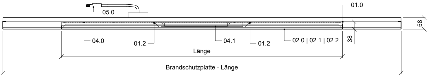
durlum dur-F30 Brandschutzplatte sep. ausgeschrieben
