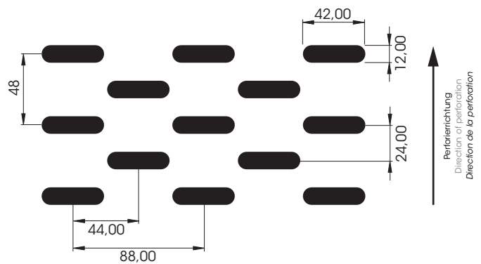
Skizze verkleinert dargestellt | Drawing is reduced in size | Croquis en dimension réduite
